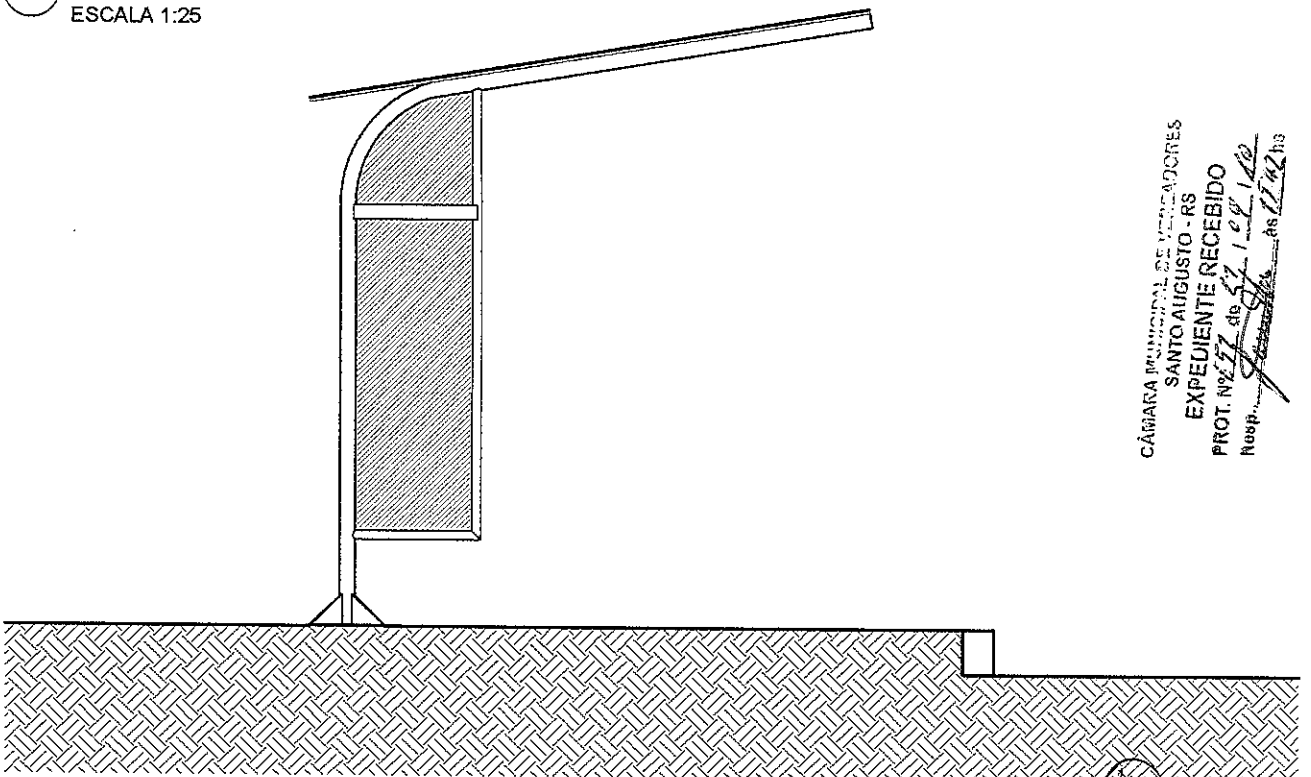
02 FACHADA ESQUERDA ESCALA 1:25
